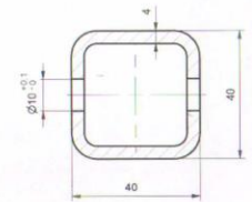
A-A (1:1)
