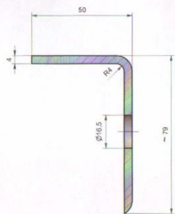
A-A (1:1)
