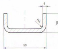
A-A (1:1)
