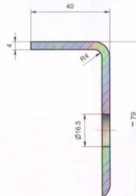
A-A (1:1)
