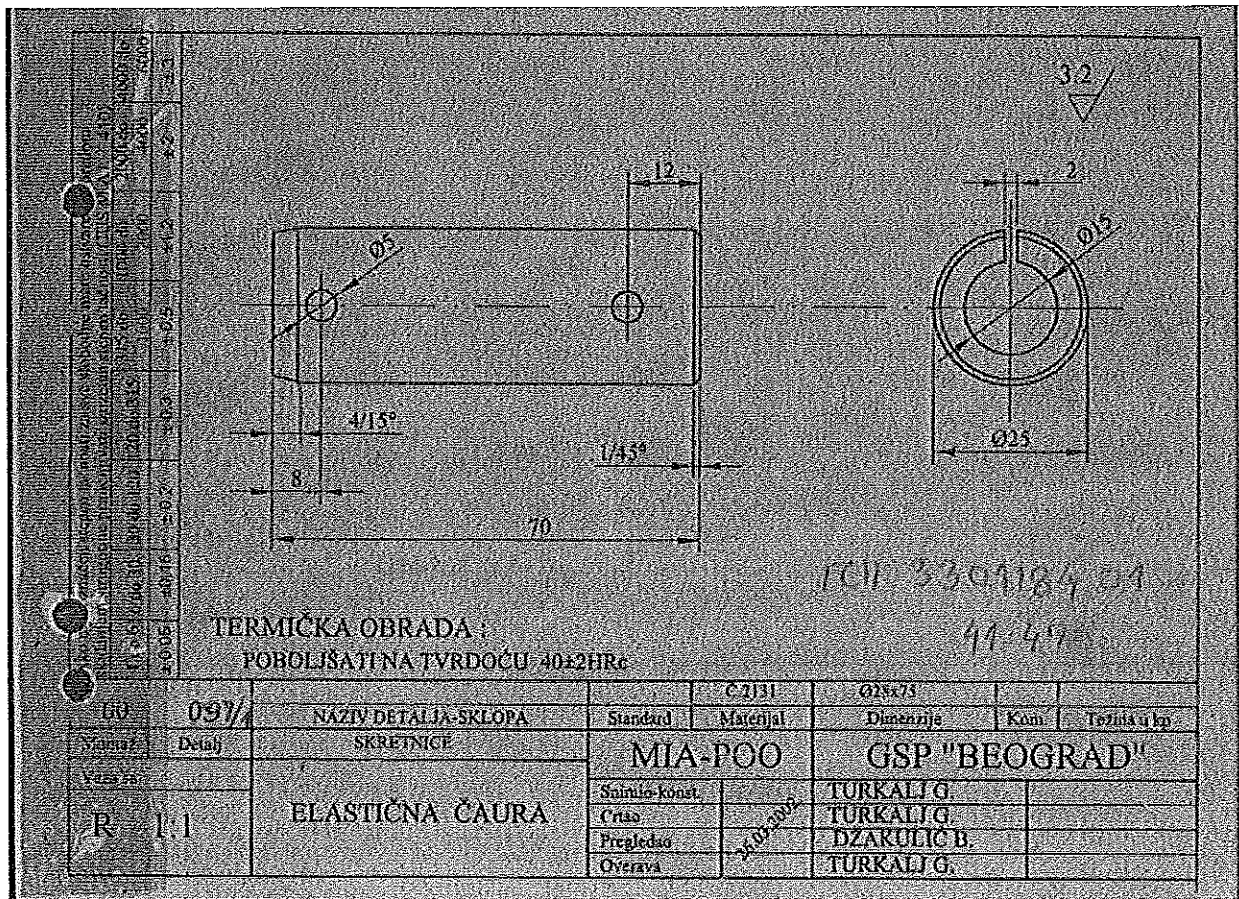
Позиција 59: цртеж - MIA-POO-00-097-1
