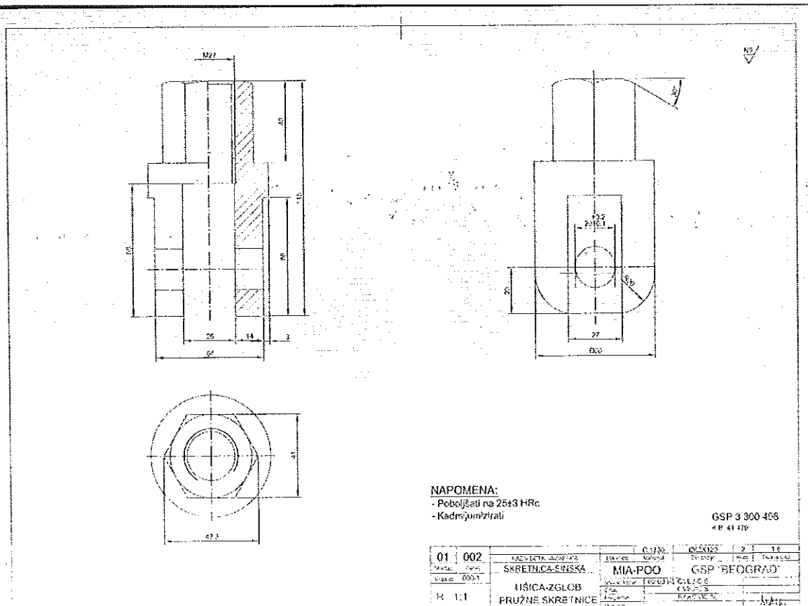
Позиција 8: цртеж - MIA-POO-01-002
