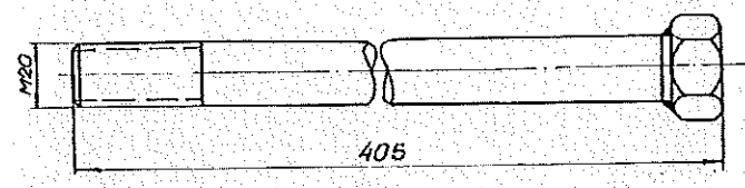
СКЛОП ЛЕЖИШТА 1
