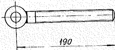
СКЛОП ВИЉУШКЕ 1
