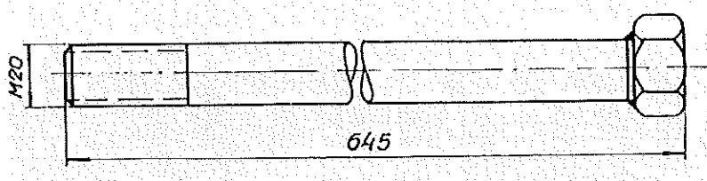
СКЛОП ОСОВИНЕ 2
