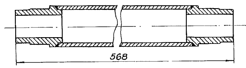
СКЛОП ЛЕЖИШТА 2
