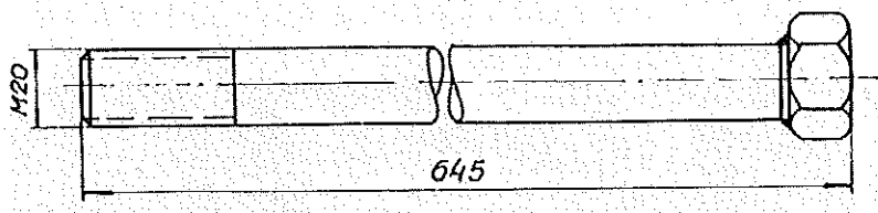
СКЛОП ОСОВИНЕ 2
