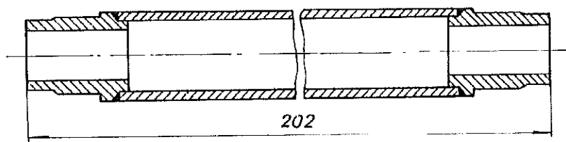
СПОЈНА ПОЛУГА
