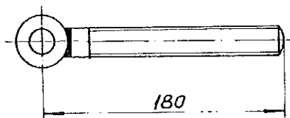
СКЛОП ЗАВРТЊА 2
