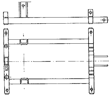
ДОЊИ РАМ
