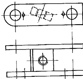
СКЛОП ВИЉУШКЕ 2
