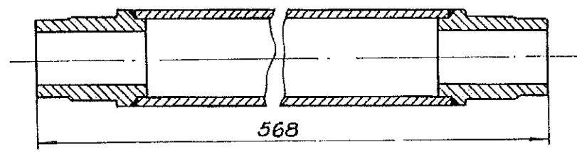
СКЛОП ЛЕЖИШТА 2
